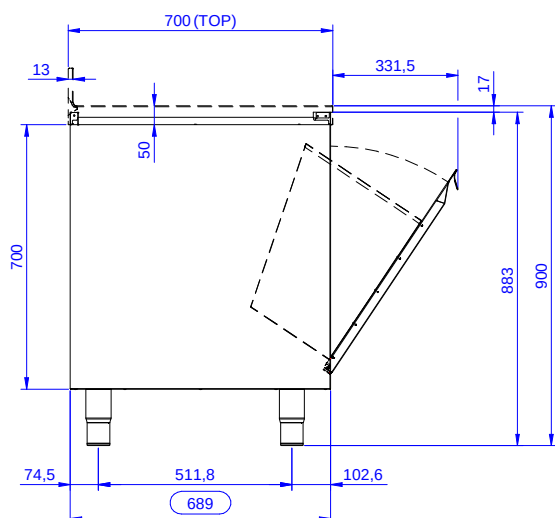
Oldalnézet
